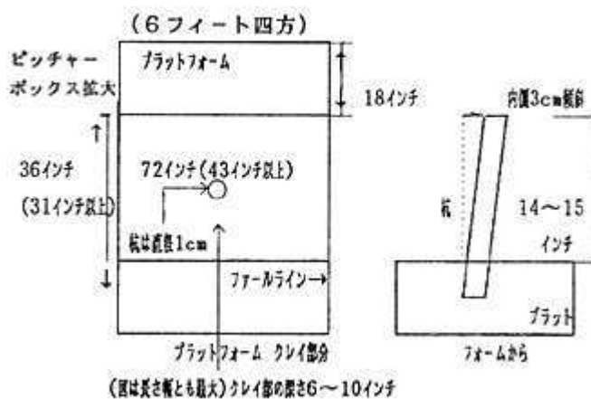
寸法規格は図のとおり
