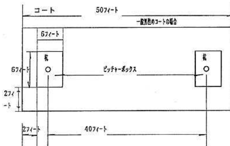
寸法規格は図のとおり
